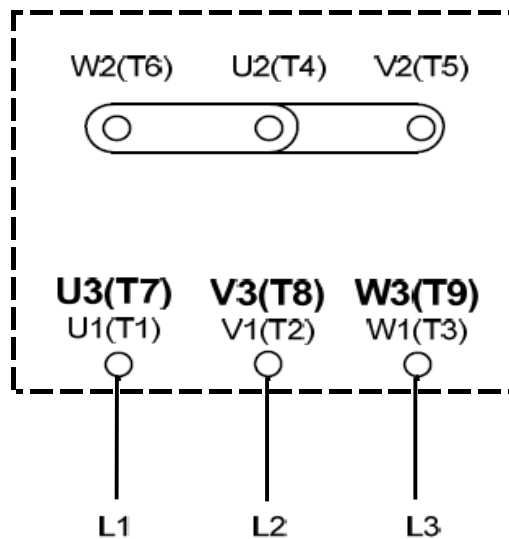
ALIMENTACIÓN ELÉCTRICA
