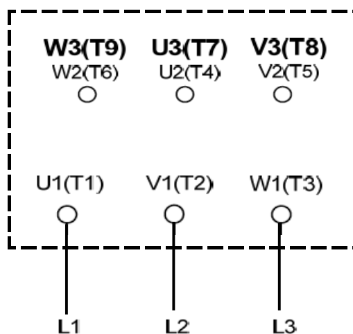
ALIMENTACIÓN ELÉCTRICA
